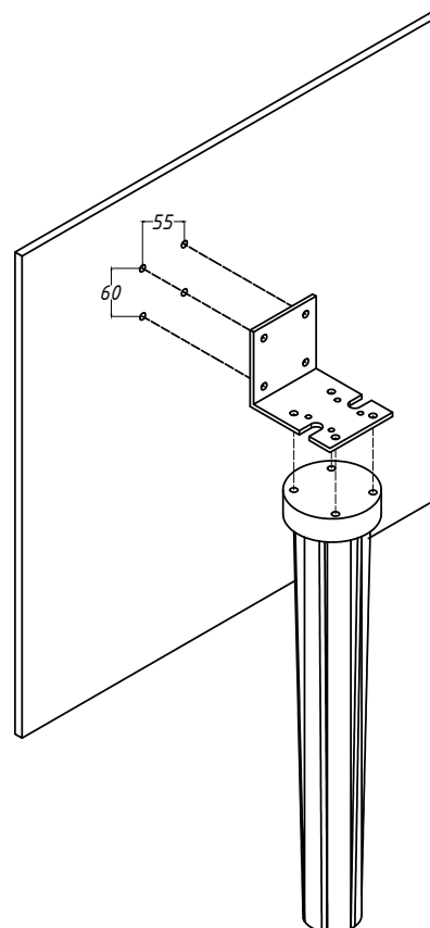
Рисунок 12 Крепление модулей фильтров.
