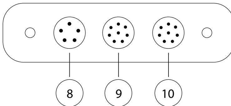
Рисунок 15 Панель электрических входов/выходов центрально модуля увлажнения.
