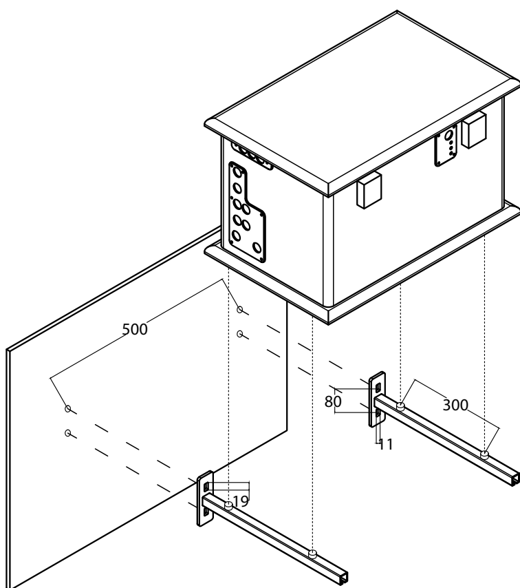
Рисунок 11 Схема монтажа центрального модуля системы увлажнения Buhler -AHS M12UV.
