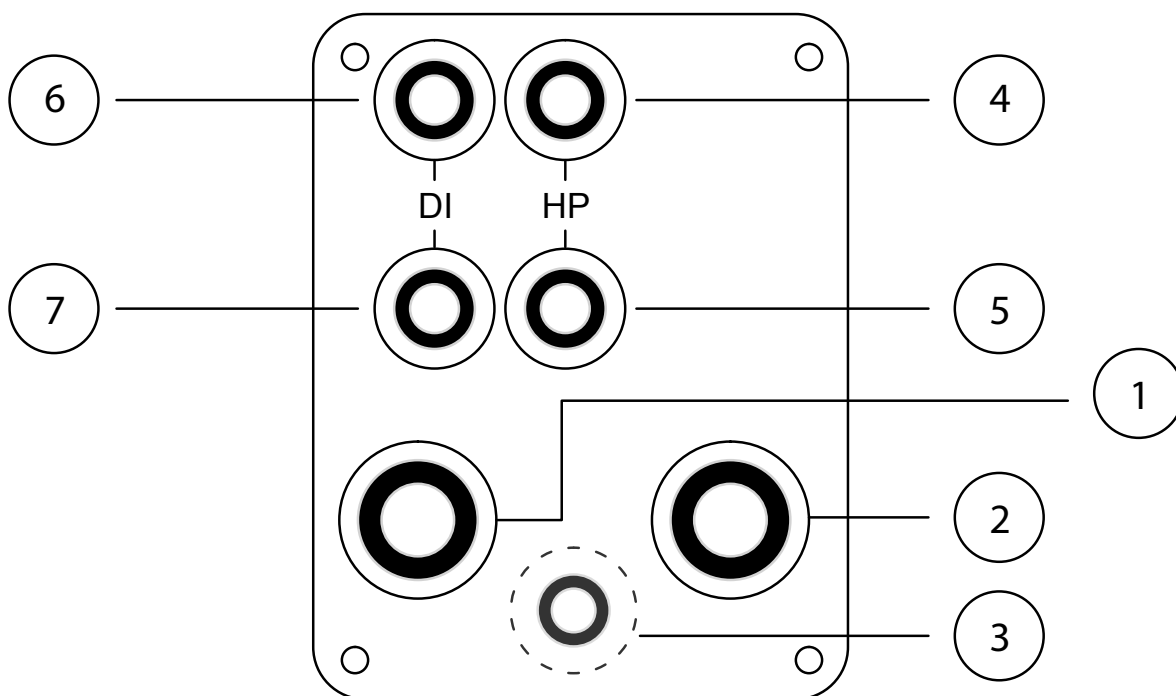
Рисунок 14 Панель гидравлических входов/выходов центрального блока увлажнения.
