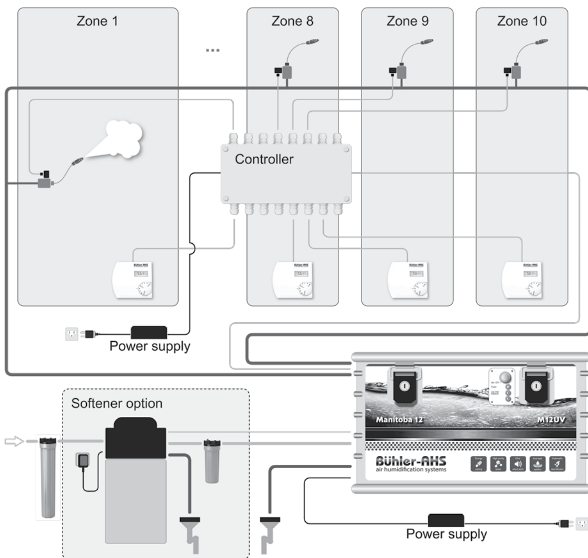
Рисунок 1 Структурная схема адиабатической системы увлажнения Buhler-AHS Manitoba 12.
