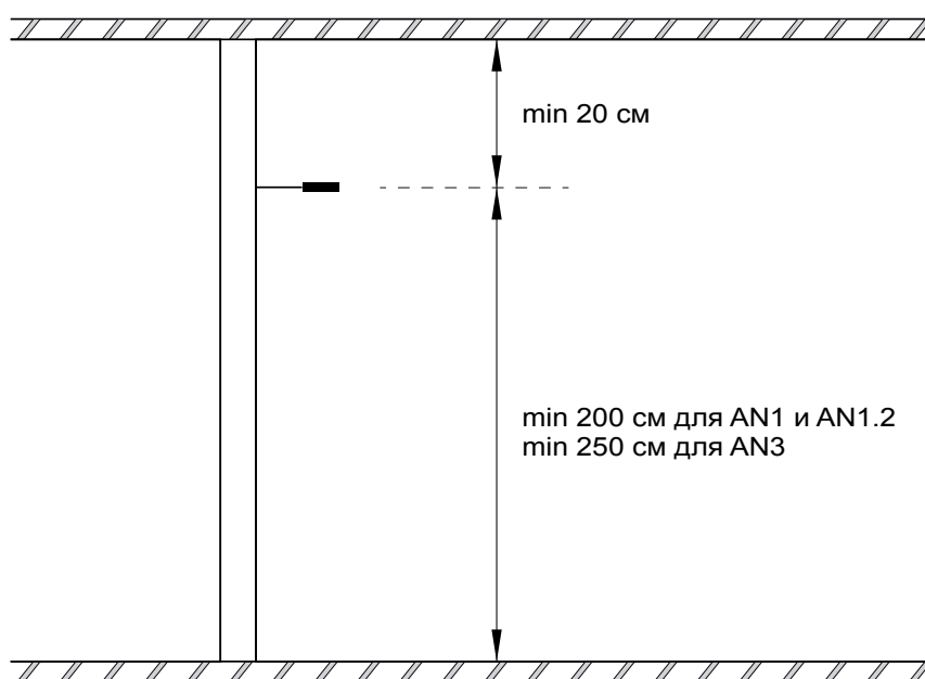
Рисунок 17 Положение распыляющей форсунки.
